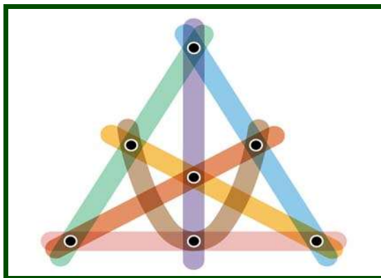
شکل ۳: دومین ابرگراف اکسترمال
