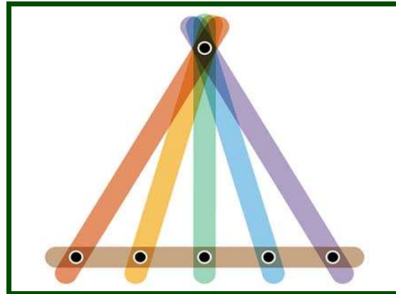
شکل ۴: سومین ابرگراف اکسترمال
