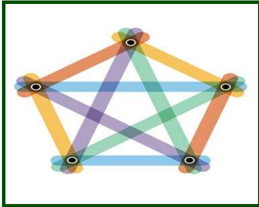
شکل ۲: اولین ابرگراف اکسترمال (گراف کامل)
